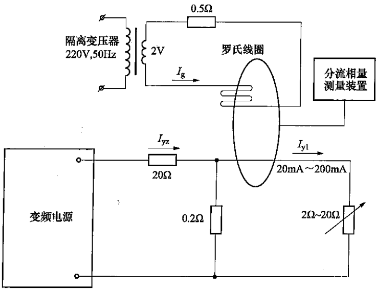
图 C.4 分流相量测量抗工频干扰电流测试
